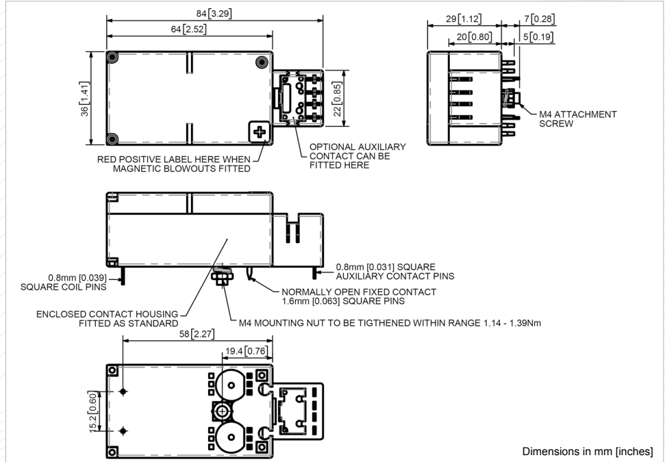
PC60
